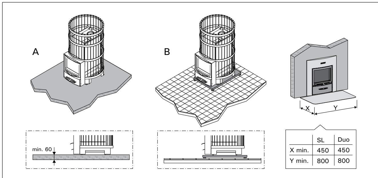
Рисунок 8. Защита пола (все размеры приведены в миллиметрах)
