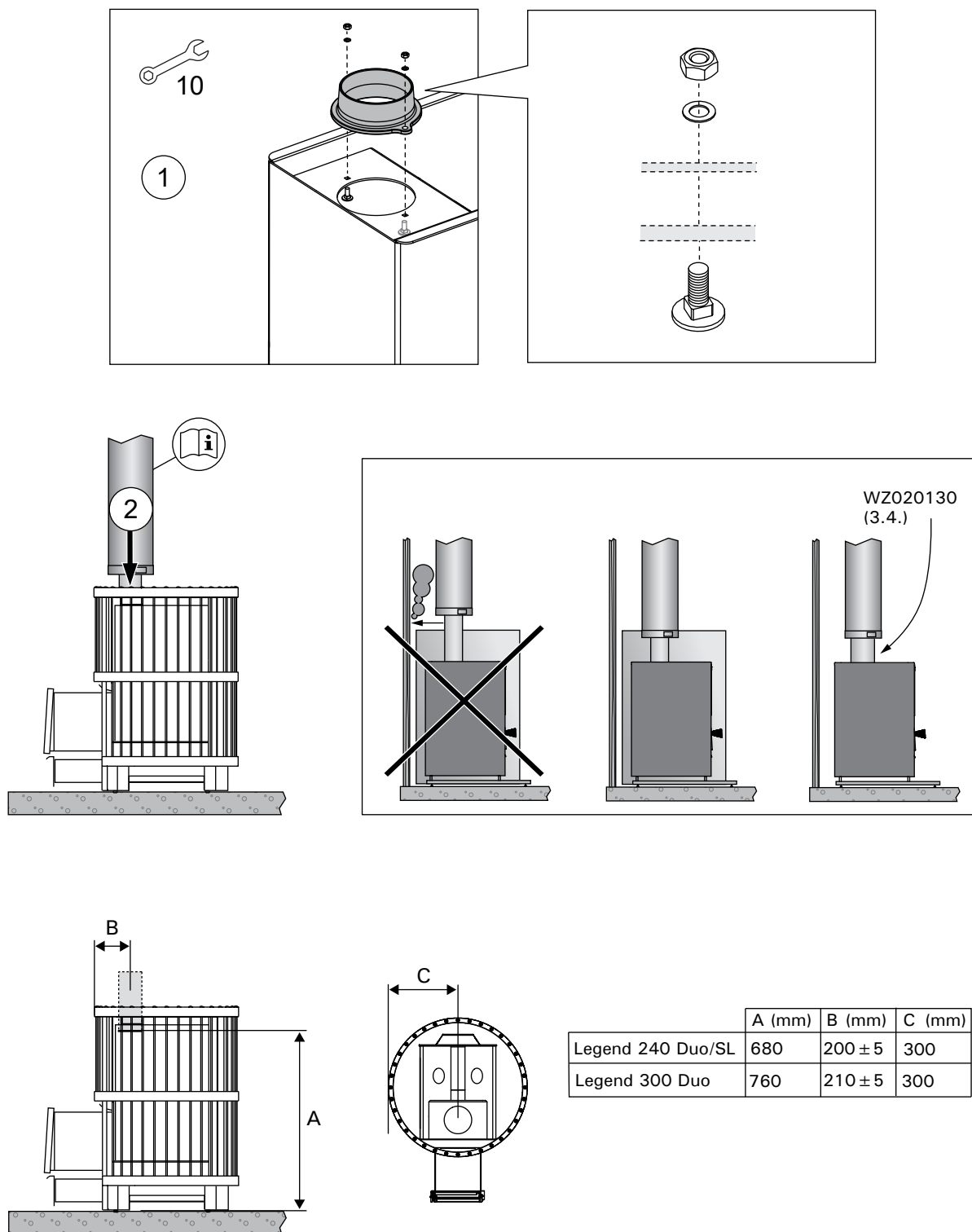
Рисунок 11. Присоединение печи к стальному дымоходу Harvia Joonis 11. Kõrse ühendamine Harvia teraskorstnaga
