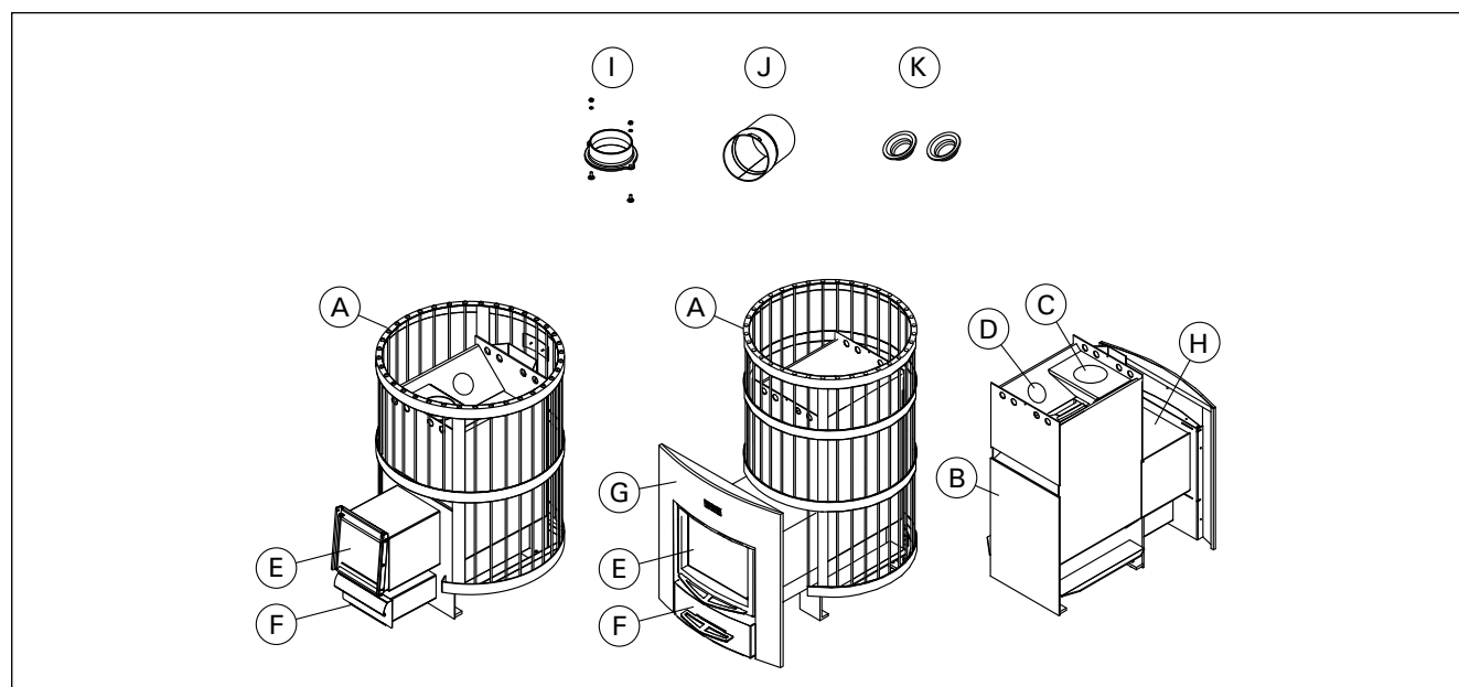
Figure 1. Composants du poêle. Toute modification du poêle sans autorisation est interdite.
