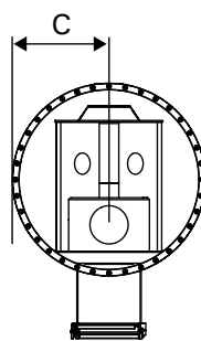
Kuva 11. Raccordement du poêle à une cheminée en acier Harvia Bild 11. Collegare la stufa a una cappa in acciaio Harvia
