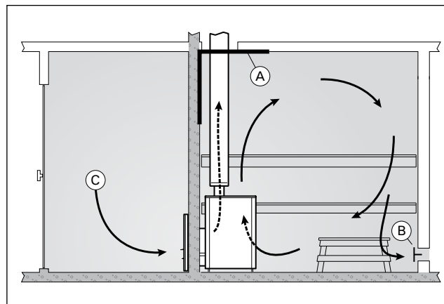
Figure 7. Mechanical exhaust ventilation Abbildung 7. Mechanische Entlüftung
